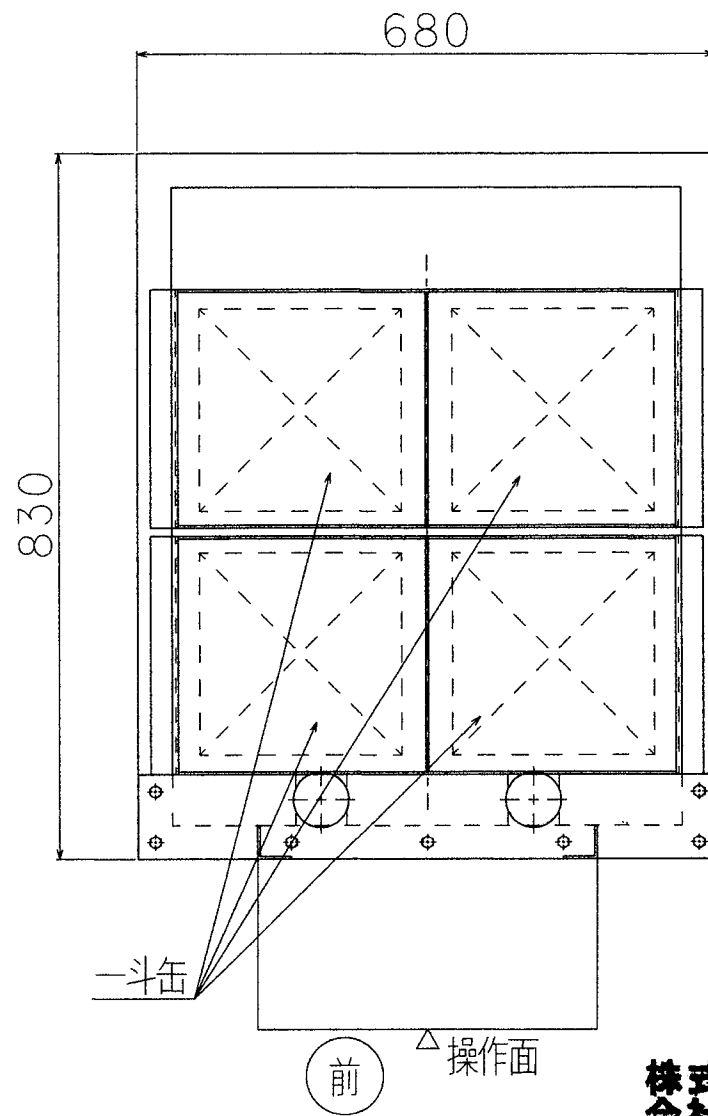
電気ヒータ式湯煎槽 (寸法改訂)
