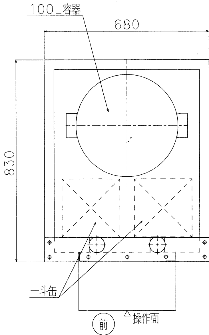
電気ヒータ式湯煎槽 (寸法改訂)
