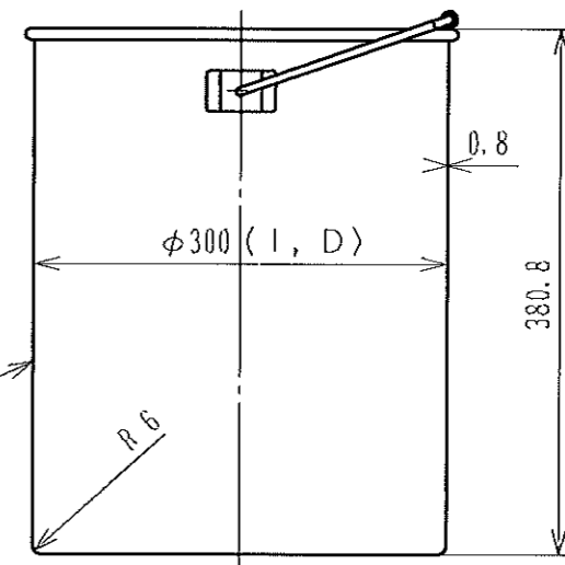
内容器 容量約 26L
